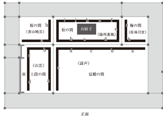
唐招提寺御影堂平面図
